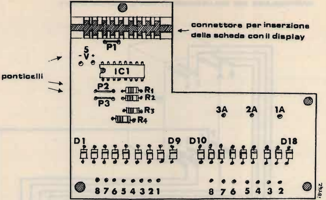
LAYOUT DEI COMPONENTI
