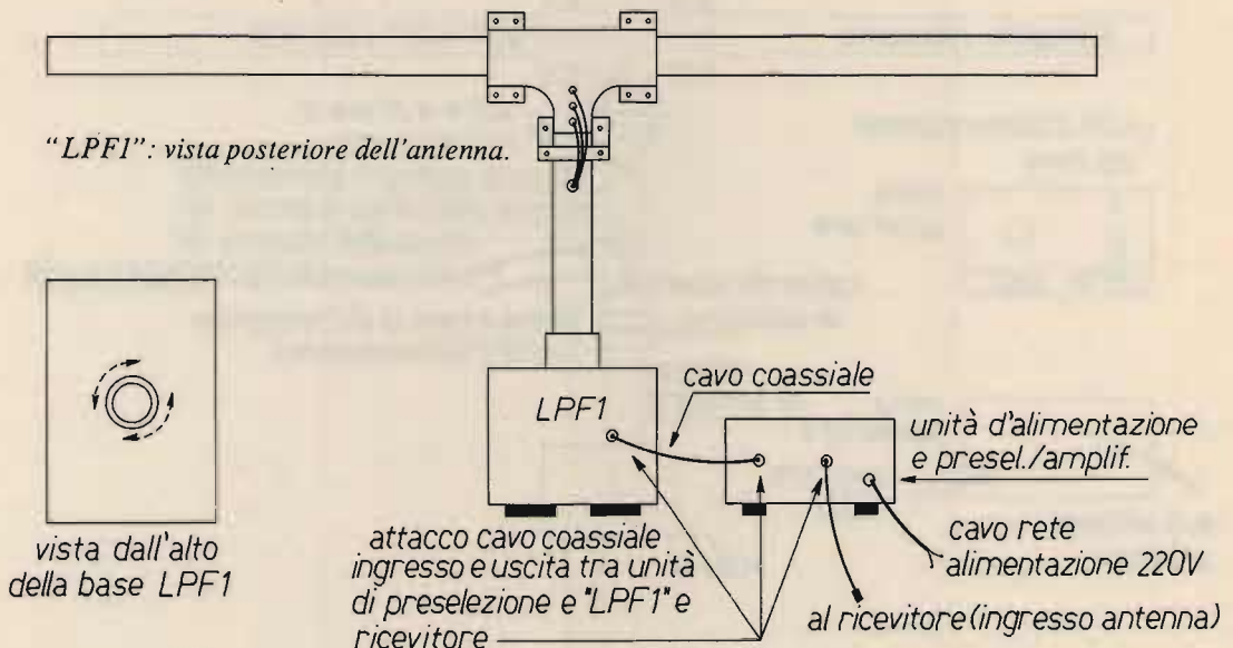
Esemplificazione delle connessioni tra "LPF1", unità di alimentazione da rete (preselezione e amplificazione) e ricevitore.
