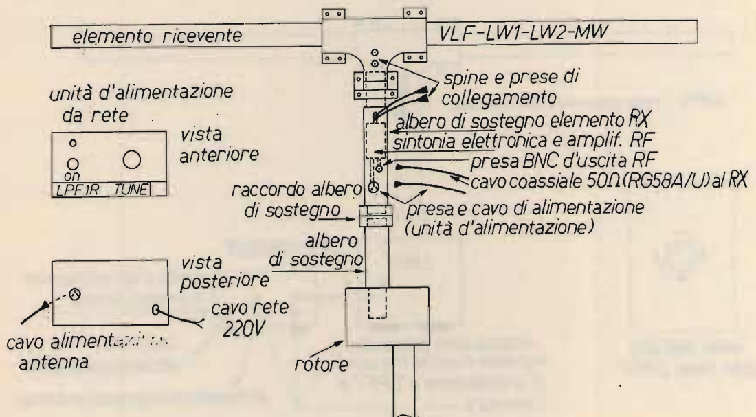
Esemplificazione installazione e connessioni antenna "LPF1 - R" (controllo remoto).
