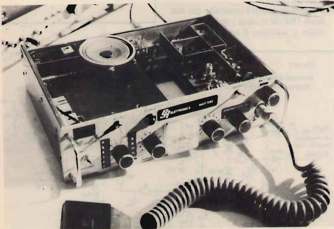
Il prototipo ultimato e completo di microfono con commutazione "Push To Talk" (PTT).
