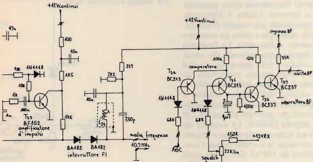
Ricetrasmittitore SSB/CW per i 2 m: noise blanker e squelch (disegno di pugno dell'Autore).
