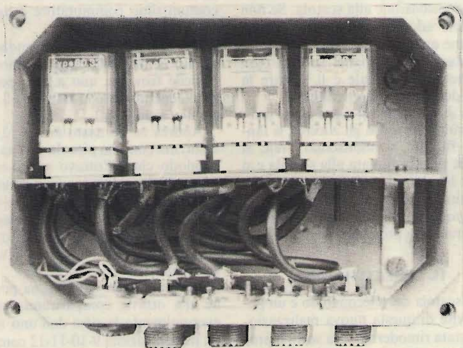
Vista interna dei relé. Quelli usati sono a tre scambi (uno non è usato). In basso si può ben vedere la filatura con lo RG-58 e il collegamento comune di massa.
